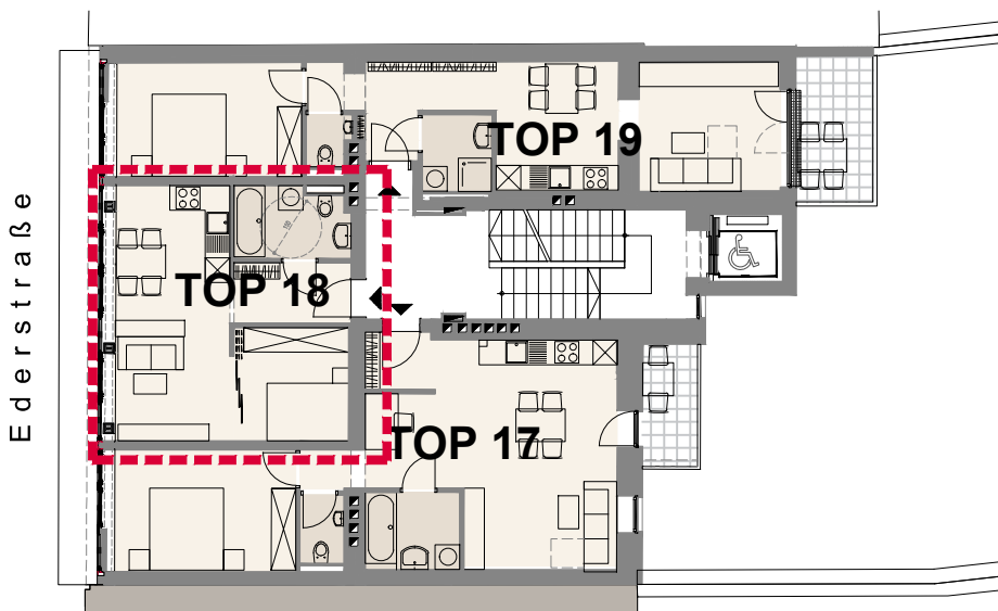
ÜBERSICHT Geschoß M 1:200
